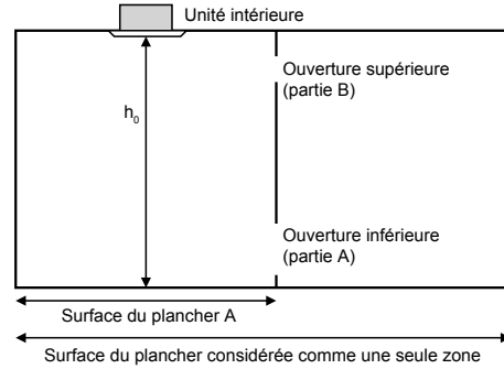
Exemple de calcul de l'Anv min (h 0 = 2,2 m)
