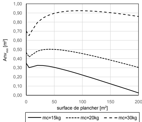
Exemple de calcul de l'Anv min (h 0 = 1,8 m)
