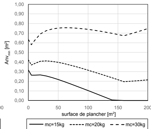
Exemple de calcul de l'Anv min (h 0 = 2,2 m)
