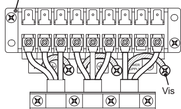
Câble de raccordement (Unité A) Câble de raccordement (Unité B) Cordon d'alimentation
