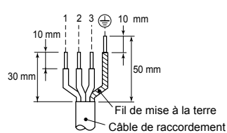
Câblage d'alimentation pour plusieurs unités intérieures
