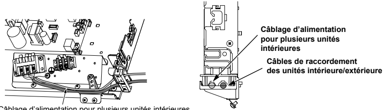
Câblage d'alimentation pour plusieurs unités intérieures
