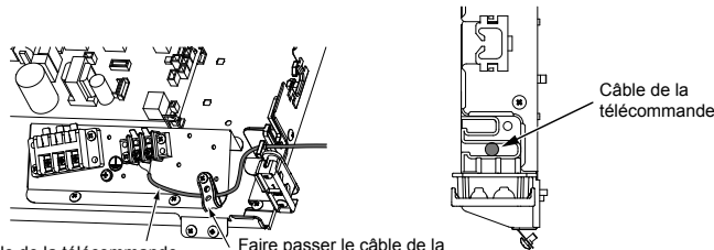
Câble de la télécommande
