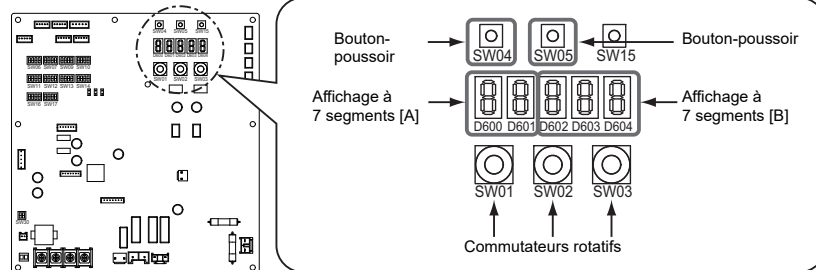
Carte de circuits imprimés de l'interface
