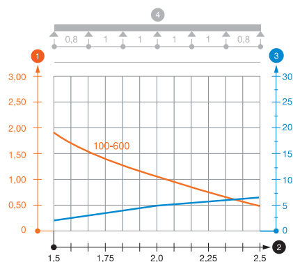
Diagramme de charge du chemin de câbles MKSMU 85
