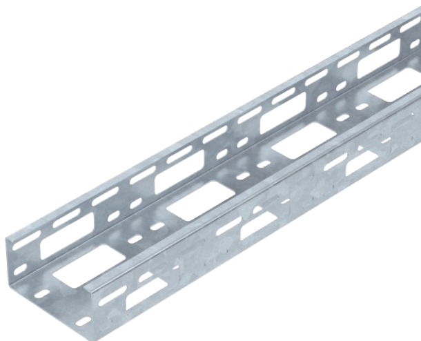
Canal AZ d'une hauteur d'aile de 50 mm.
