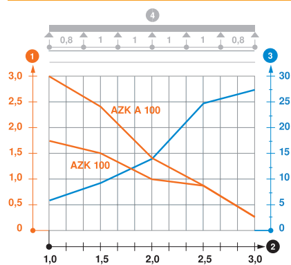
Diagramme de charge du canal AZ
