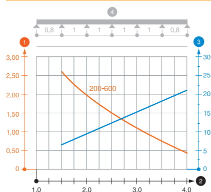
Diagramme de charge LG 60 NS
