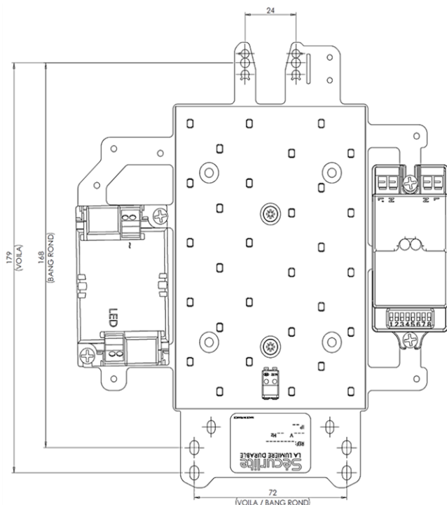
Platine avec détecteur :
