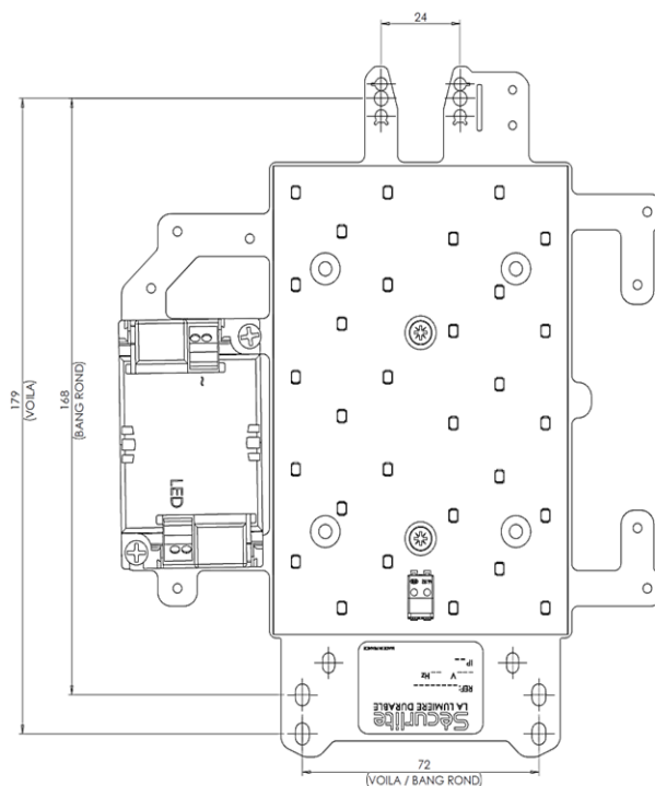
Platine sans détecteur :
