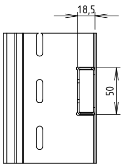
COUPE B-B ECHELLE 1 : 4
