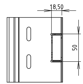
COUPE B-B ECHELLE 1 : 4
