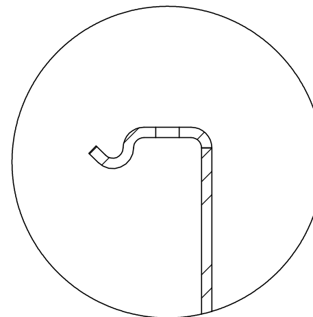
DÉTAIL D ECHELLE 2 : 1
