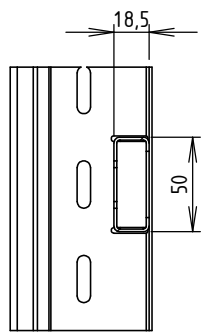
COUPE B-B ECHELLE 1 : 4
