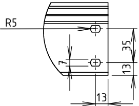
DÉTAIL A ECHELLE 1 : 4
