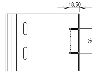
COUPE B-B ECHELLE 1 : 4
