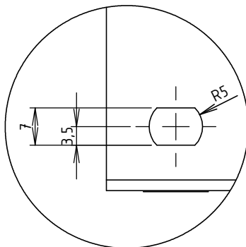
DÉTAIL A ECHELLE 1 : 1
