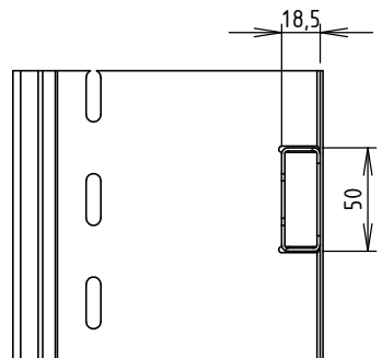
COUPE B-B ECHELLE 1 : 4
