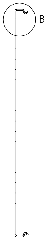
COUPE A-A ECHELLE 1 : 2
