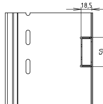
COUPE C-C ECHELLE 1 : 4
