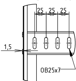
DÉTAIL C ECHELLE 1 : 5
