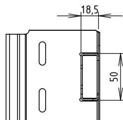
COUPE A-A ECHELLE 1 : 4
