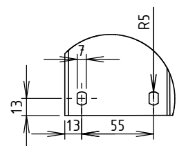
DÉTAIL D ECHELLE 1 : 4
