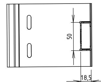
COUPE A-A ECHELLE 1 : 4
