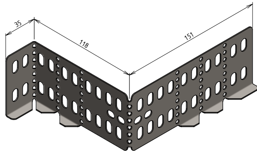
PLIAGE 120mm
