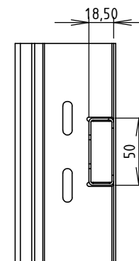
COUPE C-C ECHELLE 1 : 4
