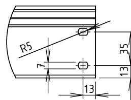
DÉTAIL A ECHELLE 1 : 4
