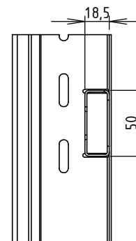
COUPE C-C ECHELLE 1 : 4
