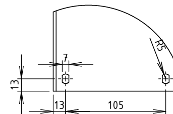
DÉTAIL D ECHELLE 1 : 4
