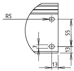
DÉTAIL A ECHELLE 1 : 4
