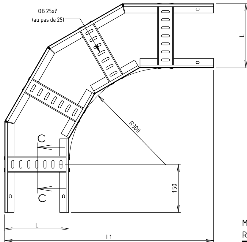
DÉTAIL A ECHELLE 1 : 4
