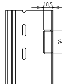
COUPE C-C ECHELLE 1 : 4
