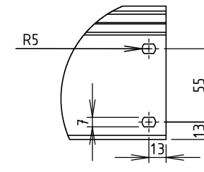
DÉTAIL A ECHELLE 1 : 4
