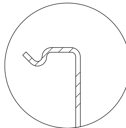
DÉTAIL B ECHELLE 2 : 1
