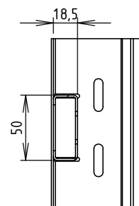
COUPE C-C ECHELLE 1 : 4
