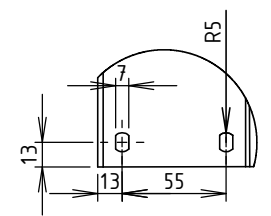
DÉTAIL D ECHELLE 1 : 4
